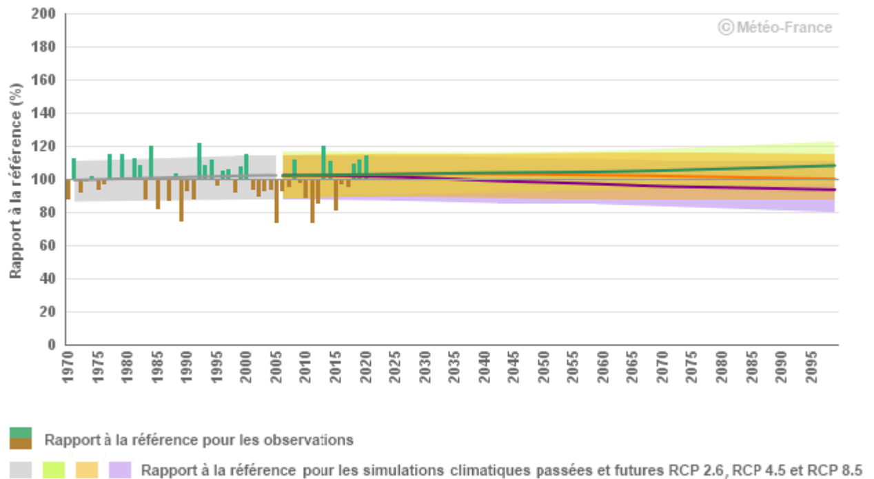
Figure 48 : Cumul annuel de précipitation en Nouvelle-Aquitaine - Simulations selon trois scénarios d'évolution
