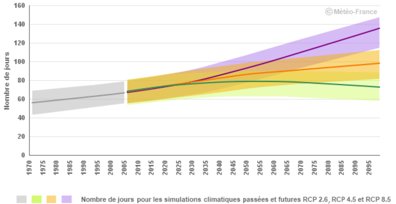
Nombre de journées chaudes en Aquitaine Simulations climatiques sur passé et futur pour trois scénarios d'évolution RCP 2.6, 4.5 et 8.5
