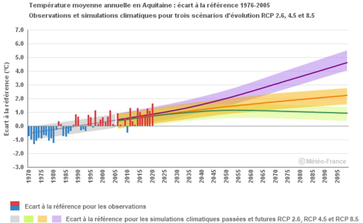
Figure 46 : Température moyenne annuelle en Nouvelle-Aquitaine - Simulations selon trois scénarios d'évolution
